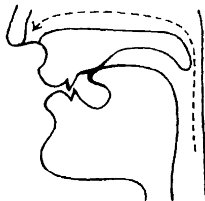
Fig. 21 /n/
