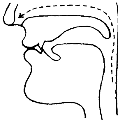
Fig. 20 /m/
