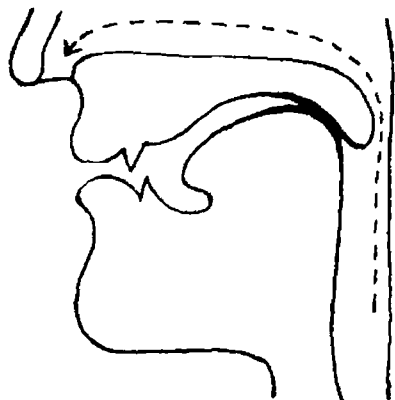
Fig. 22 /ŋ/
