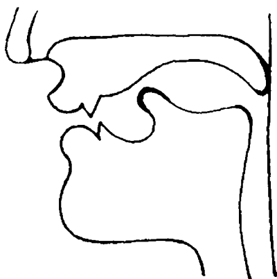
Fig. 24 /r/
